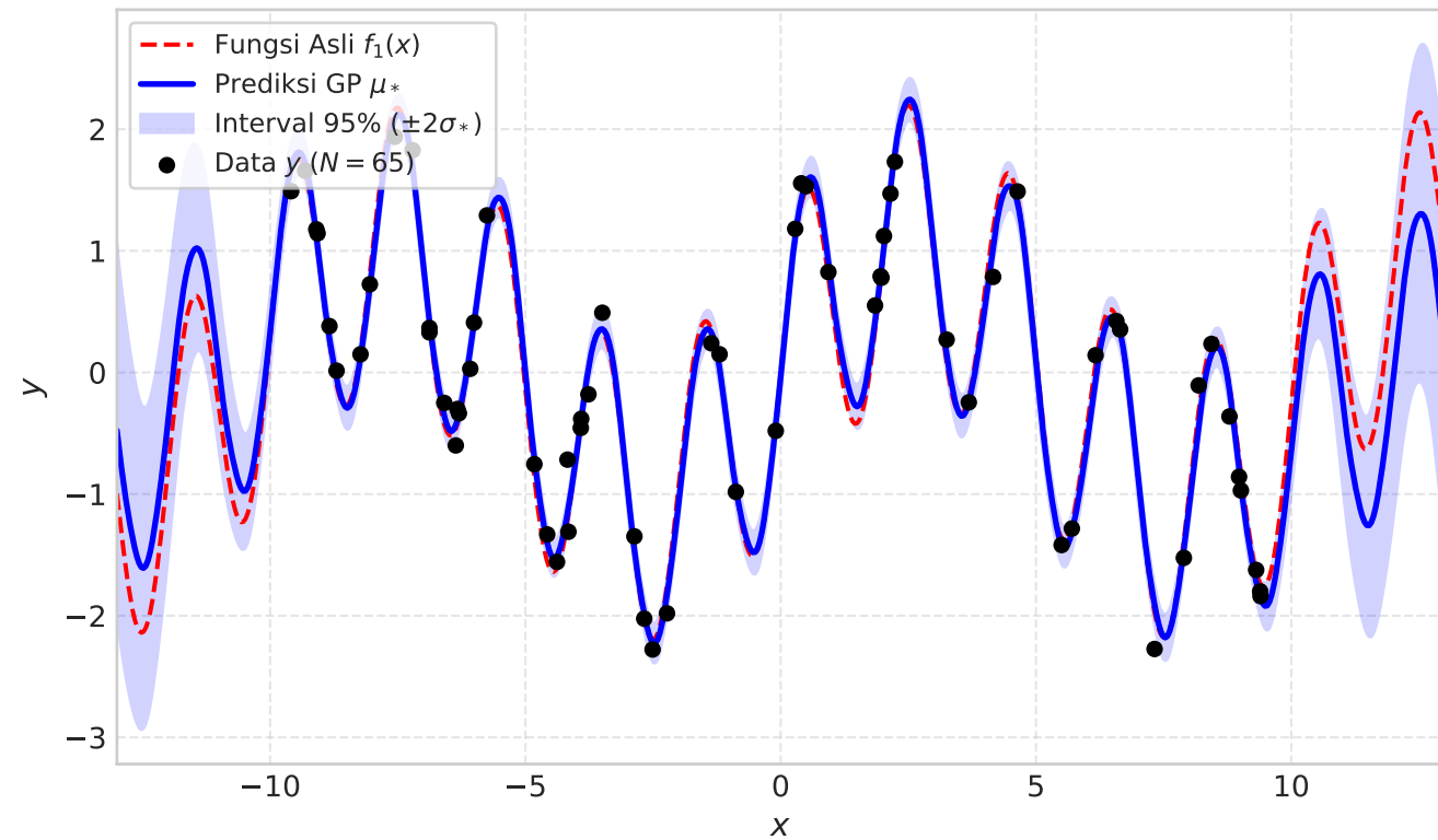
(a) Penjumlahan: k_{\text{RBF}} + k_{\text{Per}}
